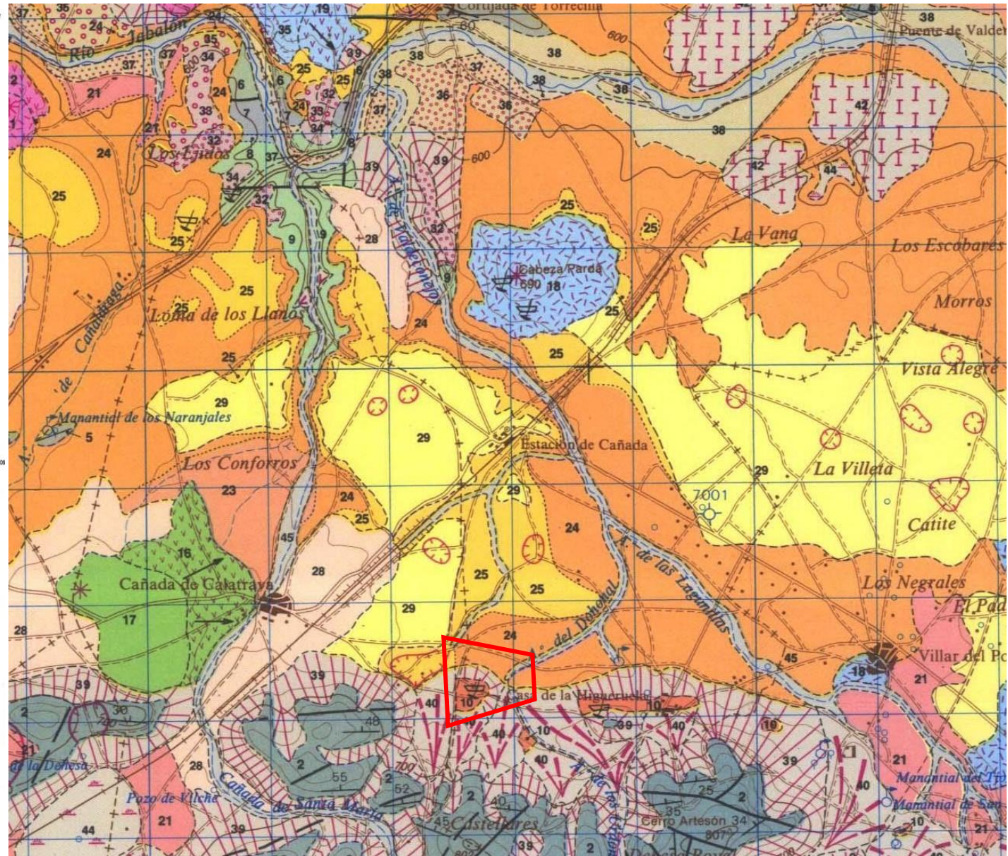
M-TM138-03 MAPA GEOLOGICO DEL LIG Costra ferro-manganesífera de casas de la Higuera. Mapa Geológico MAGNA, hoja 784 Ciudad Real. Portero et al. (1985).
