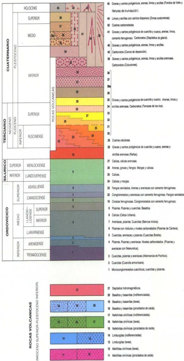
M-TM138-03 MAPA GEOLOGICO DEL LIG Costra ferro-manganesífera de casas de la Higuera. Mapa Geológico MAGNA, hoja 784 Ciudad Real. Portero et al. (1985).
